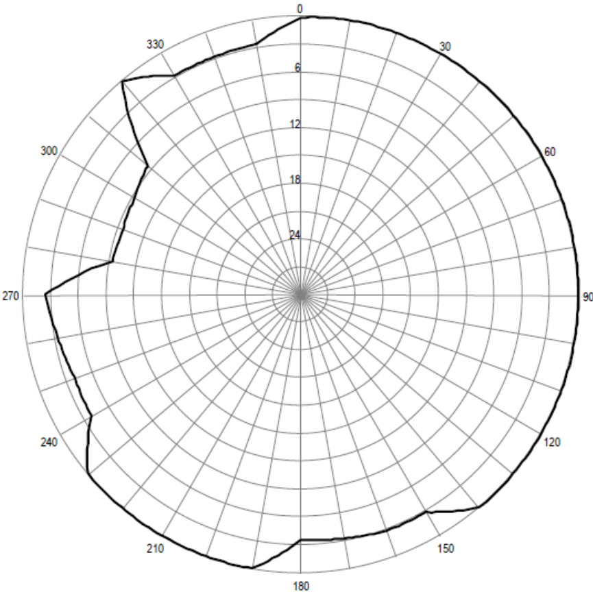
Pozioma charakterystyka promieniowania anteny stacji Warszawa Varso 104,40 MHz
